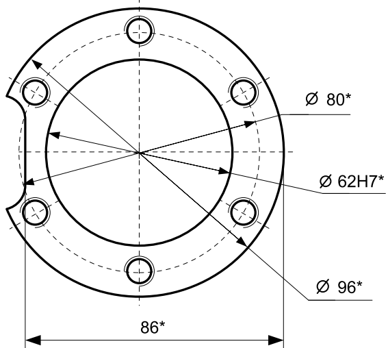
А Крышка поз. 6 условно не показана
