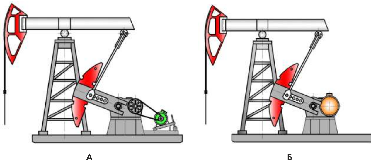
А - с традиционной клиноременной передачей, Б - с соосно установленным электродвигателем
